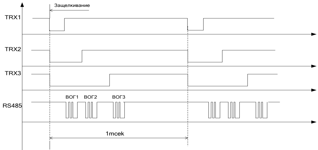
Рис.6 Пример последовательности опроса трех гироскопов.
