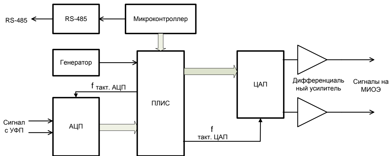
Рис.4. Структурная схема БЗО:
