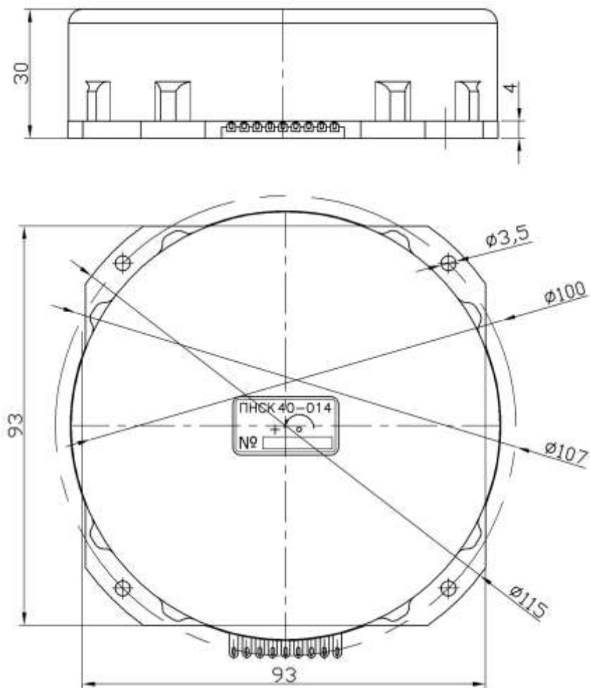
Рис.2. Габаритный чертеж прибора
