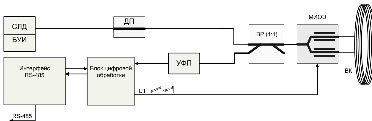
Рис.3. Структурная схема ОИУС 501:
