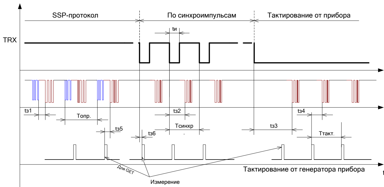
Рис.6.Временные диаграммы работы прибора
